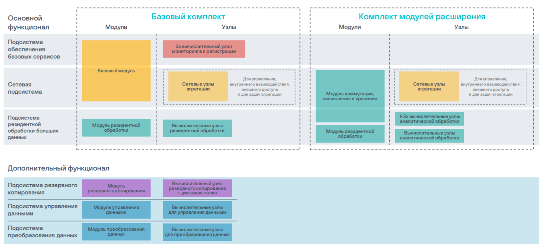
Рисунок 1. Комплектация Машины больших данных Скала^р МБД.Т
