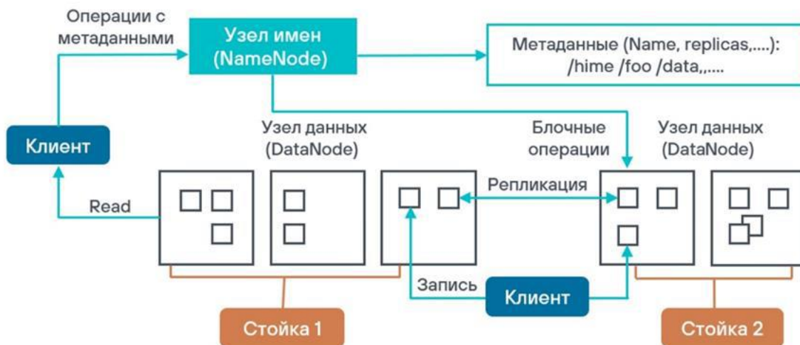
Рисунок 2. Архитектура HDFS
