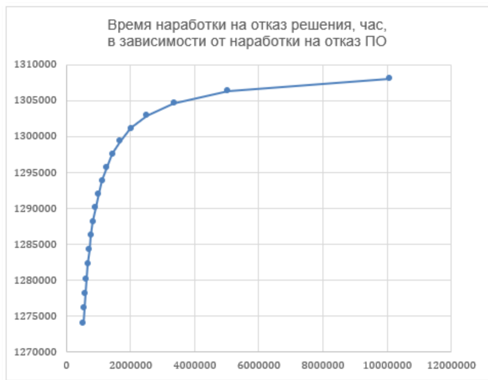
Рисунок 21. График зависимости времени наработки на отказ решения от времени наработки на отказ комплекта программного обеспечения
