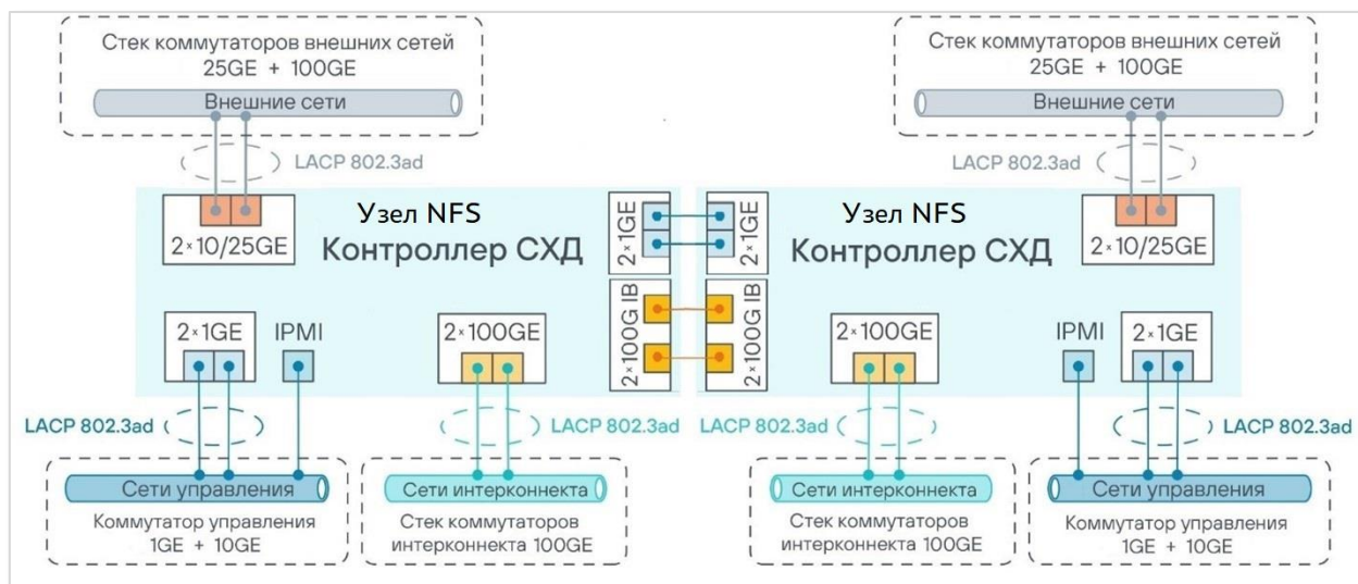
Рисунок 7. Схема сетевого взаимодействия контроллеров СХД
