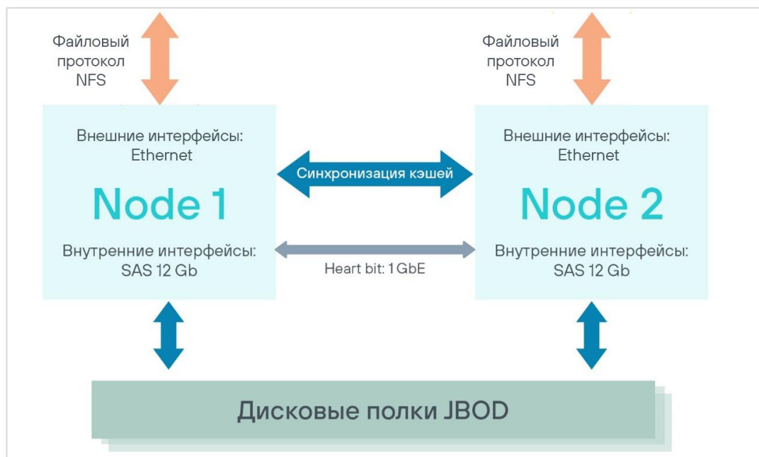
Рисунок 6. Реализация сервиса управления дисками СРК
