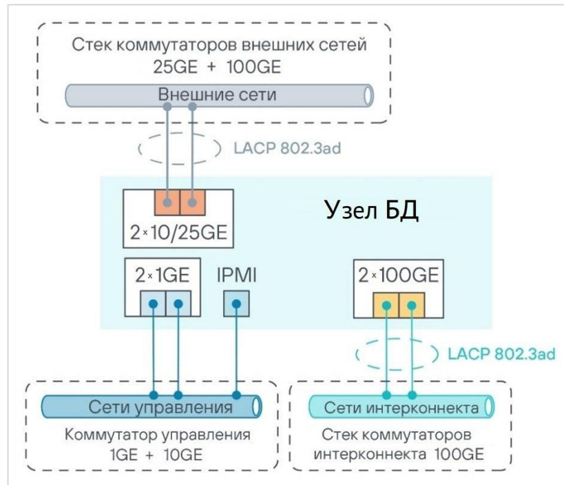
Рисунок 5. Схема сетевого взаимодействия вычислительного узла
