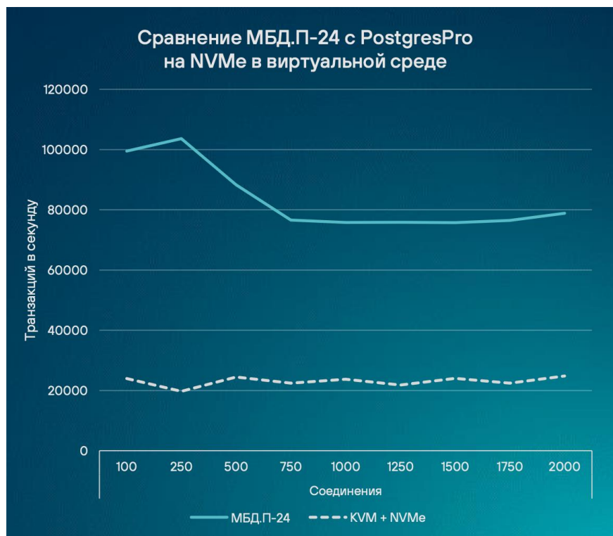
Рисунок 18. Скорость обработки запросов Машины баз данных Скала Λ р МБД.П по результатам теста pgbench
