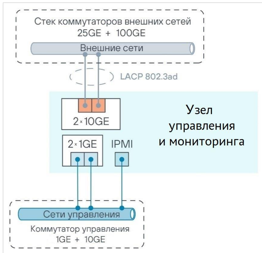
Рисунок 11. Схема сетевого взаимодействия узла управления
