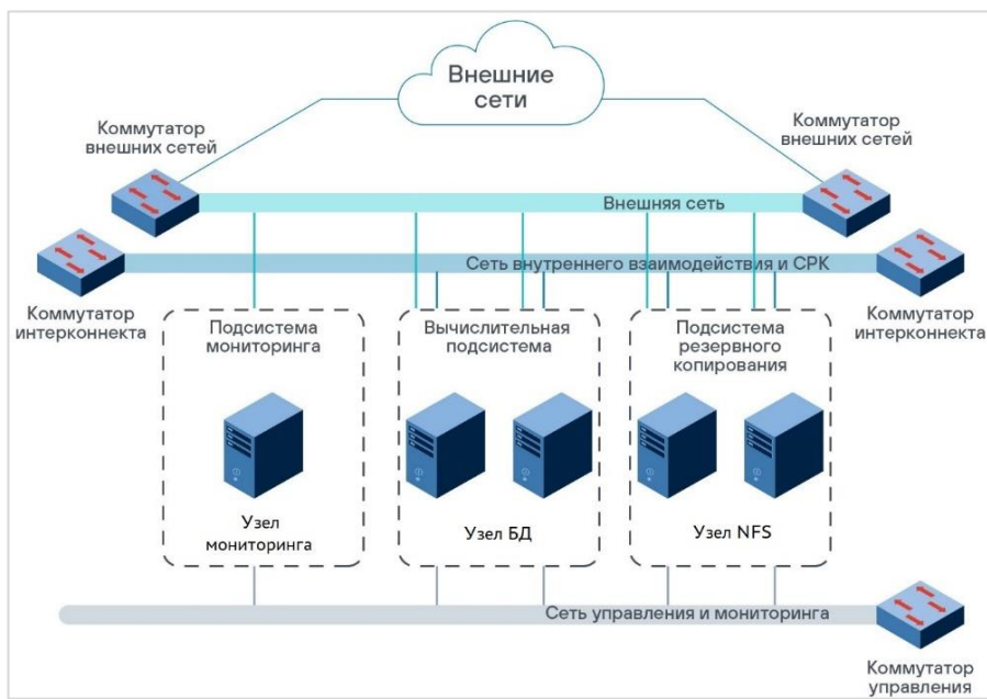
Рисунок 12. Общая схема сетевого взаимодействия
