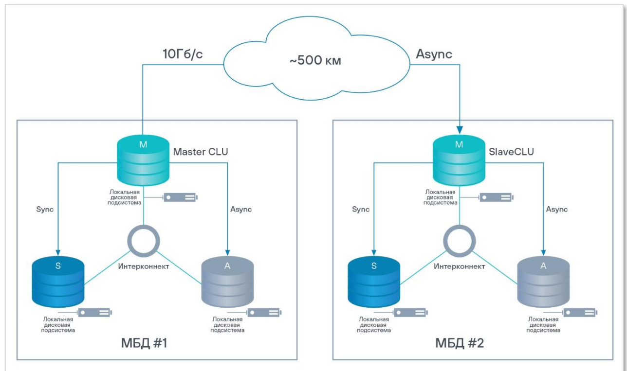
Рисунок 14. Пример реализации геокластера
