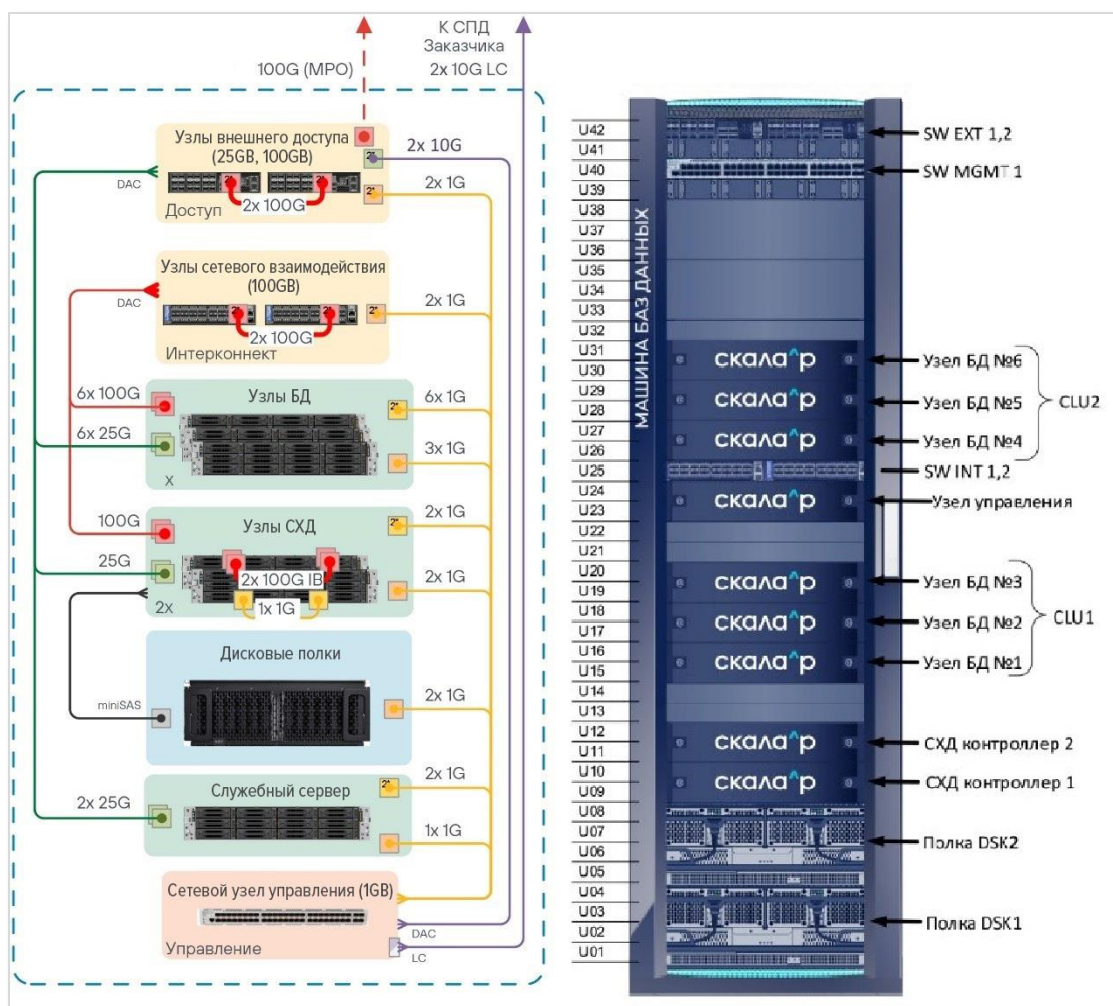
Рисунок 19. Схема взаимодействия для расчета надежности Машины баз данных Скала А р МБД.П
