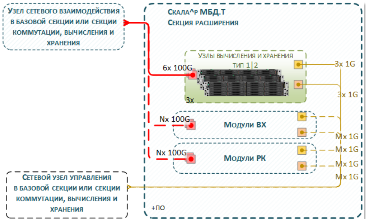
Рис. 16. Секция расширения
