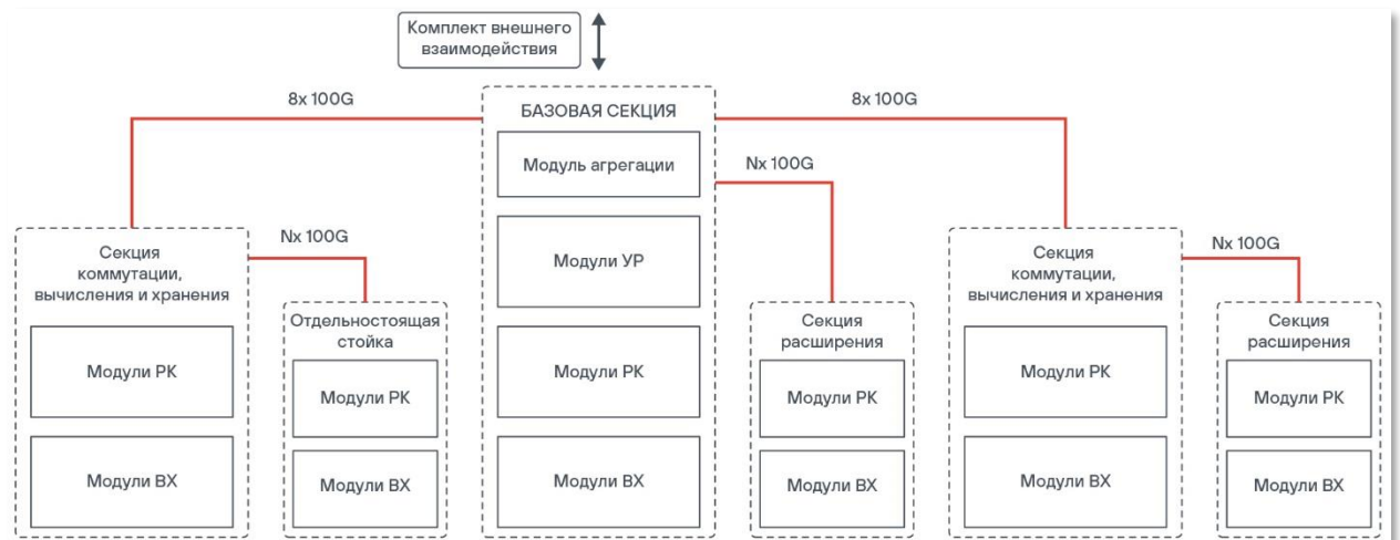
Рис. 13. Секции решения Скала Ар МБД.Т
