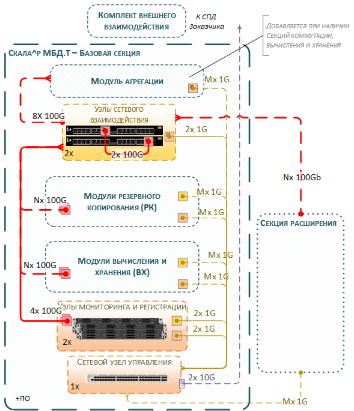
Рис. 14. Базовая секция
