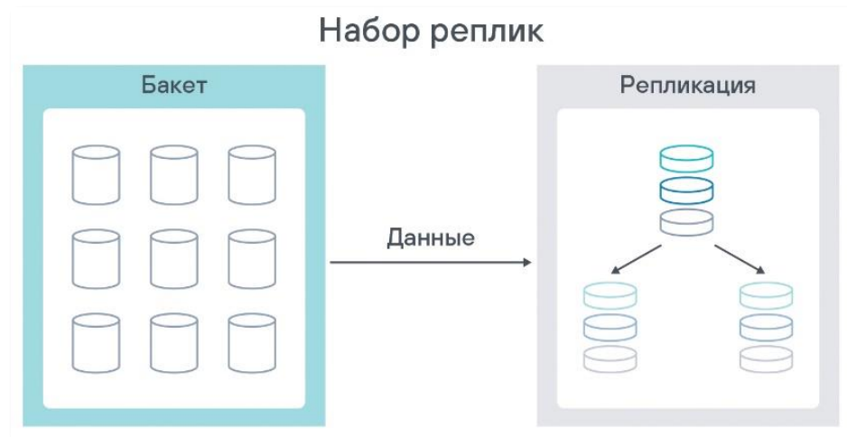
Рис. 8. Хранение данных
