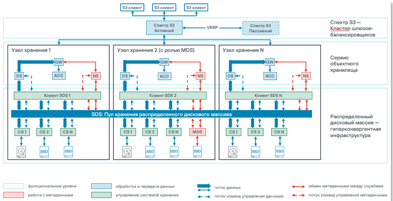
Рисунок 2. Архитектура Машины хранения данных (Схема внутренней коммутации)
