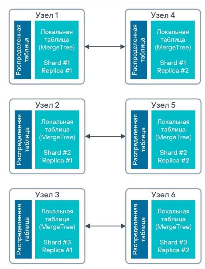
Рис. 7. Архитектура кластера
