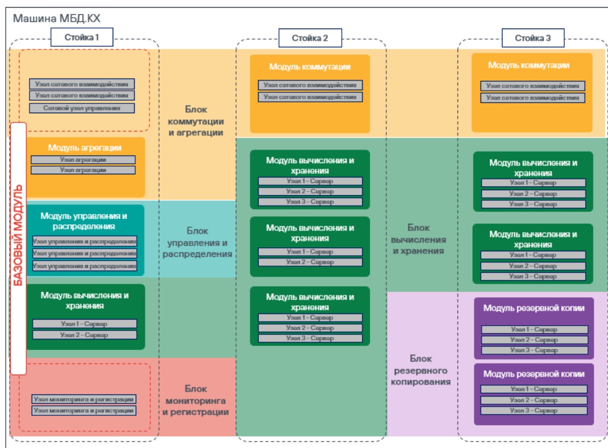
Рис. 21. Пример размещения базовых Блоков, Модулей и узлов в серверных стойках
