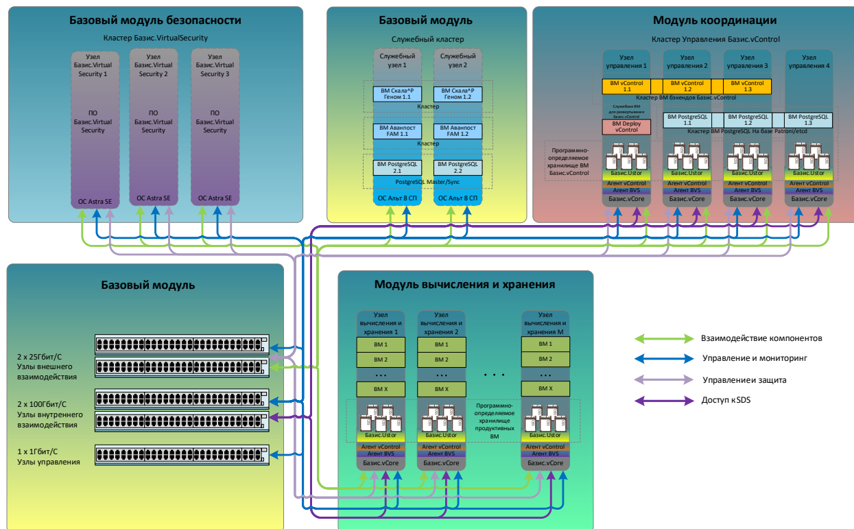
Рисунок 6. Схема исполнения 3 (максимальное исполнение ФСТЭК с SDS)
