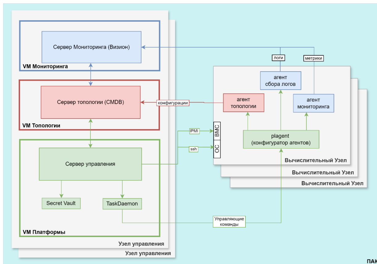
Рисунок 18. Основные компоненты программной платформы Скала^р Геном
