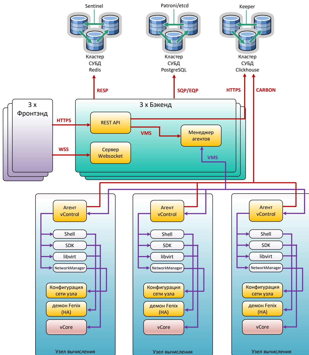
Рисунок 12. Схема взаимодействия программных компонентов ПО Базис.vControl
