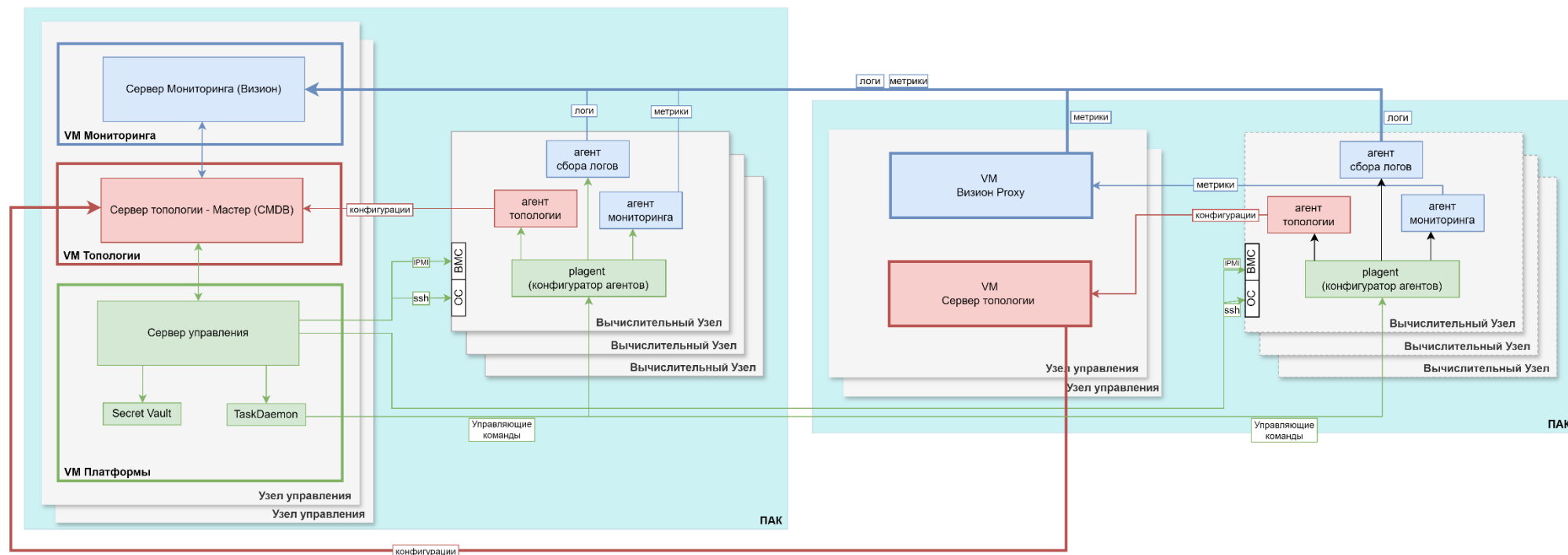
Рисунок 19. Программная платформа Скала^р Генوم в режиме централизованного управления несколькими ПАК
