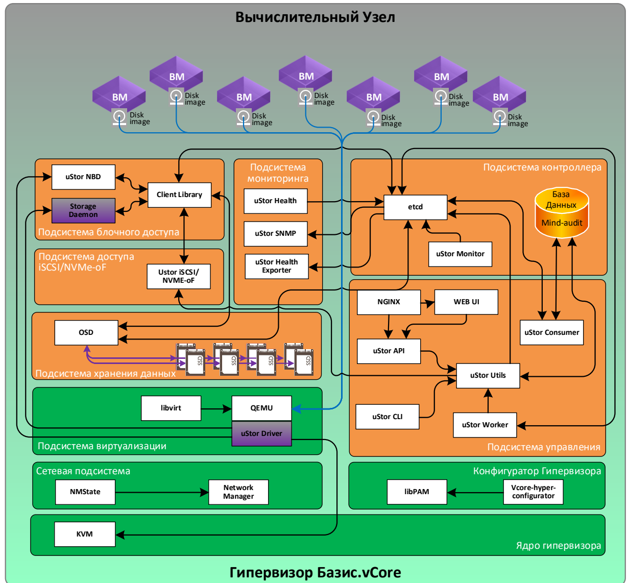
Рисунок 14. Схема взаимодействия программных компонентов программно-определяемого хранилища Базис.uStor и гипервизора Базис.vCore
