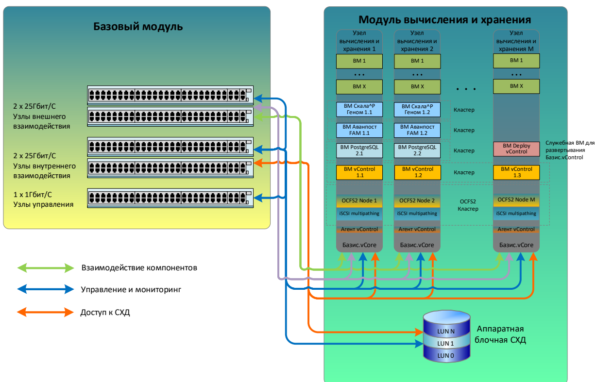
Рисунок 7. Схема исполнения 4 (минимальное исполнение с аппаратной СХД)
