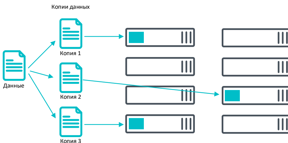
Рисунок 21. Создание реплик, полных копий данных
