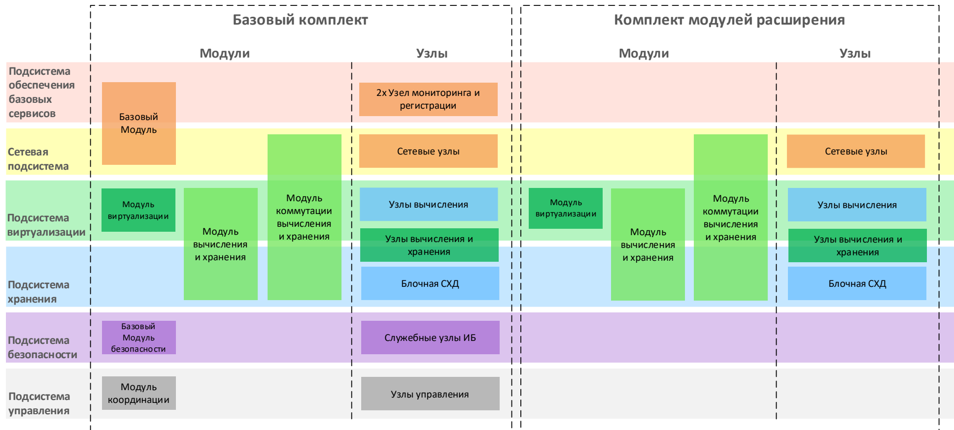
Рисунок 2. Комплектация и подсистемы Машины динамической инфраструктуры Скала^р МДИ.В
