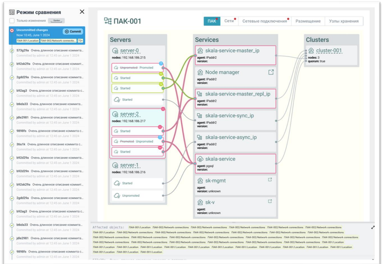
Рисунок 15. Пример интерфейса ПО Скала^р Генум (отображение схемы подключений узлов ПАК)
