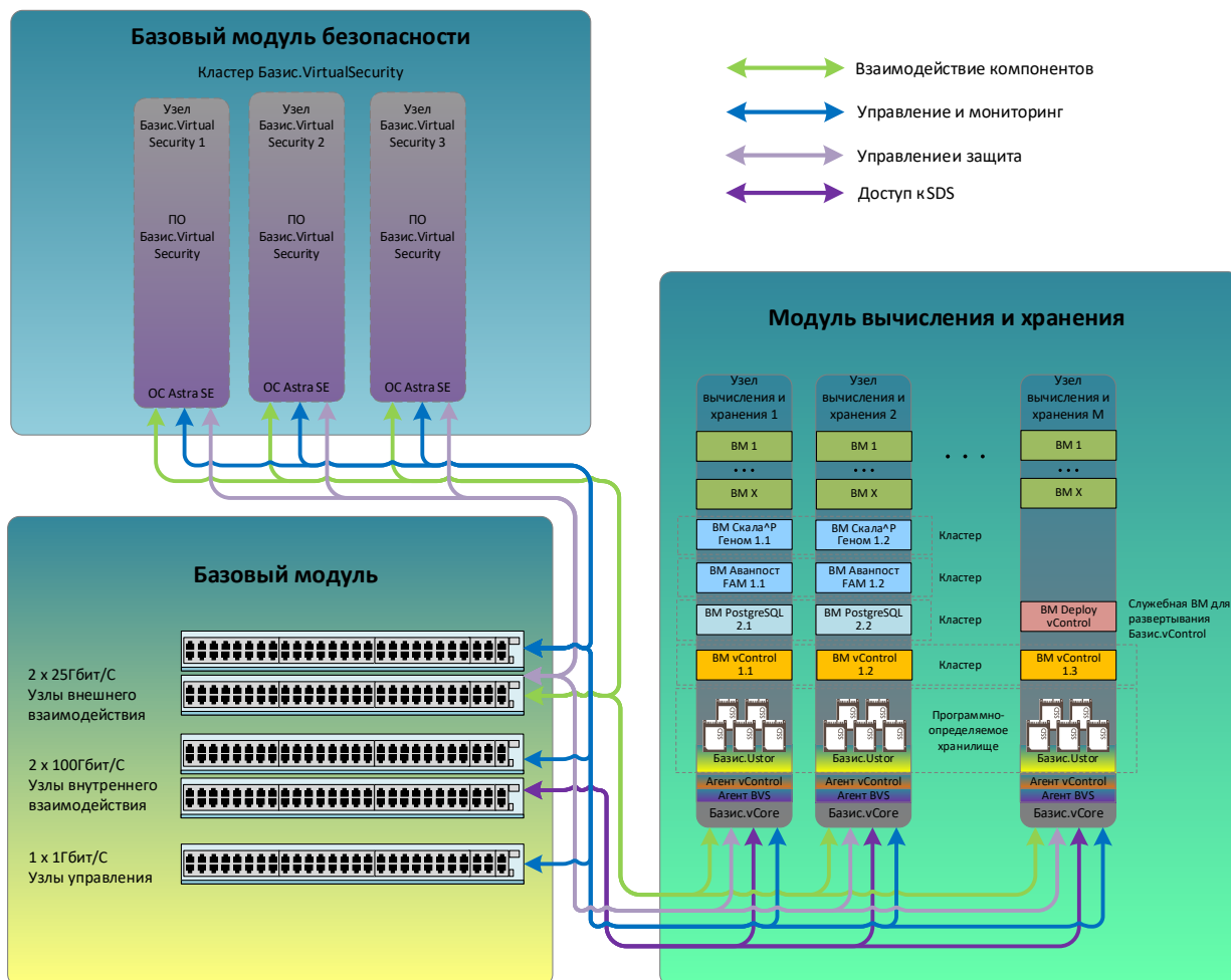
Рисунок 5. Схема исполнения 2 (минимальное исполнение ФСТЭК с SDS)
