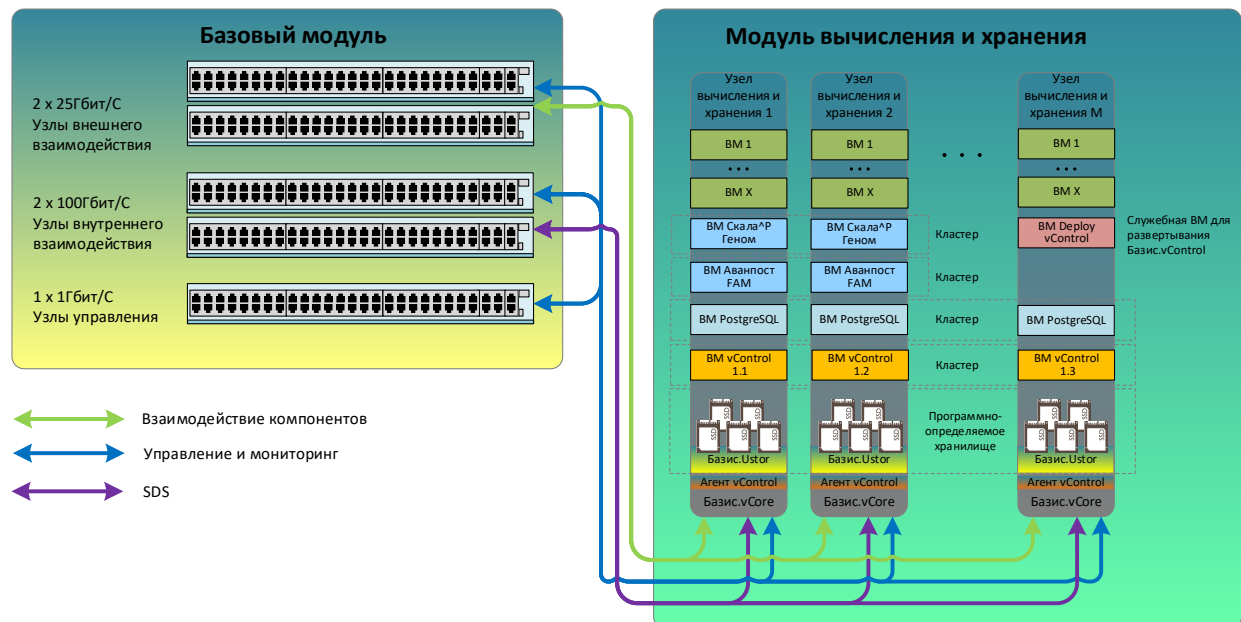
Рисунок 4. Схема исполнения 1 (минимальное исполнение с SDS)
