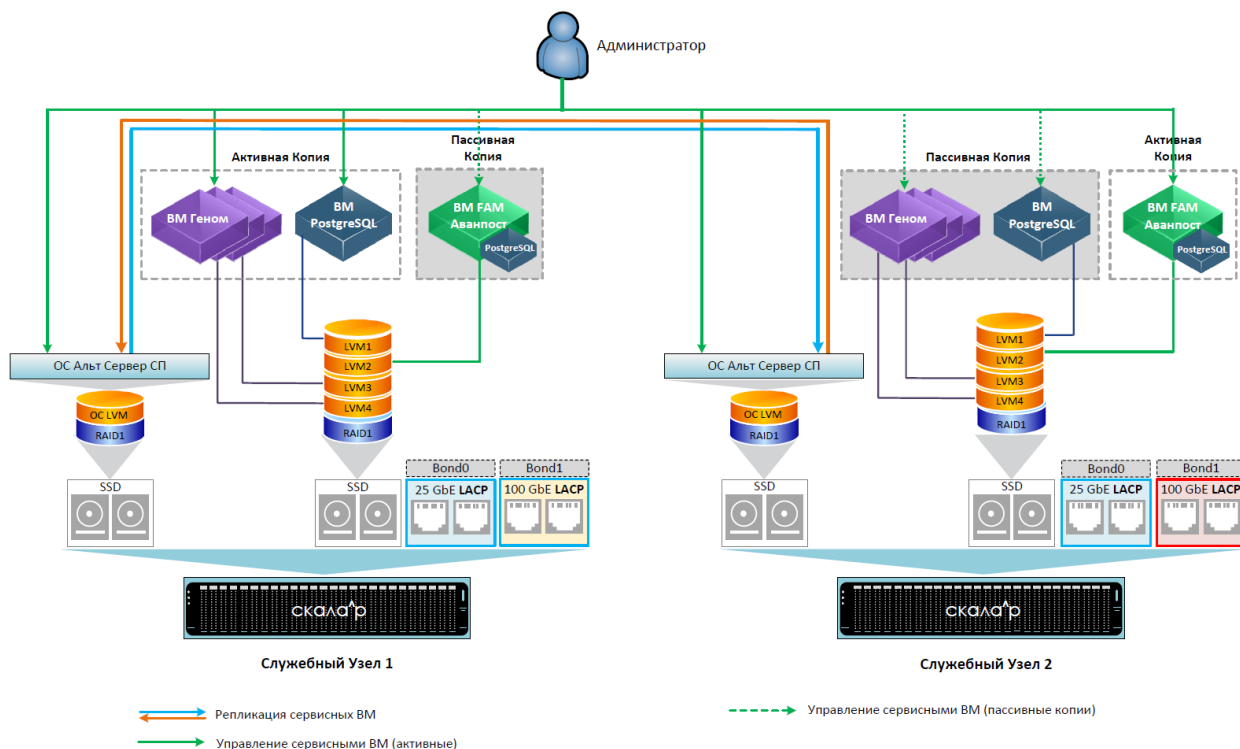
Рисунок 20. Логическая схема работы служебных узлов Скала^р МДИ.В
