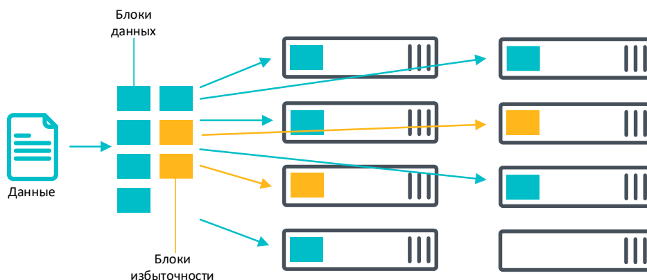
Рисунок 22. Избыточное кодирование 5 + 2
