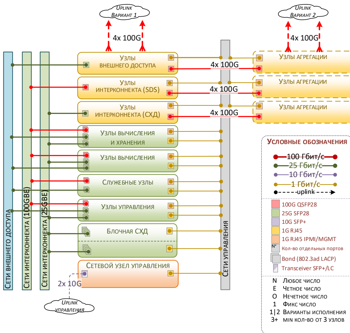
Рисунок 10. Физическая организация сетей в Машине Скала^р МДИ.В
