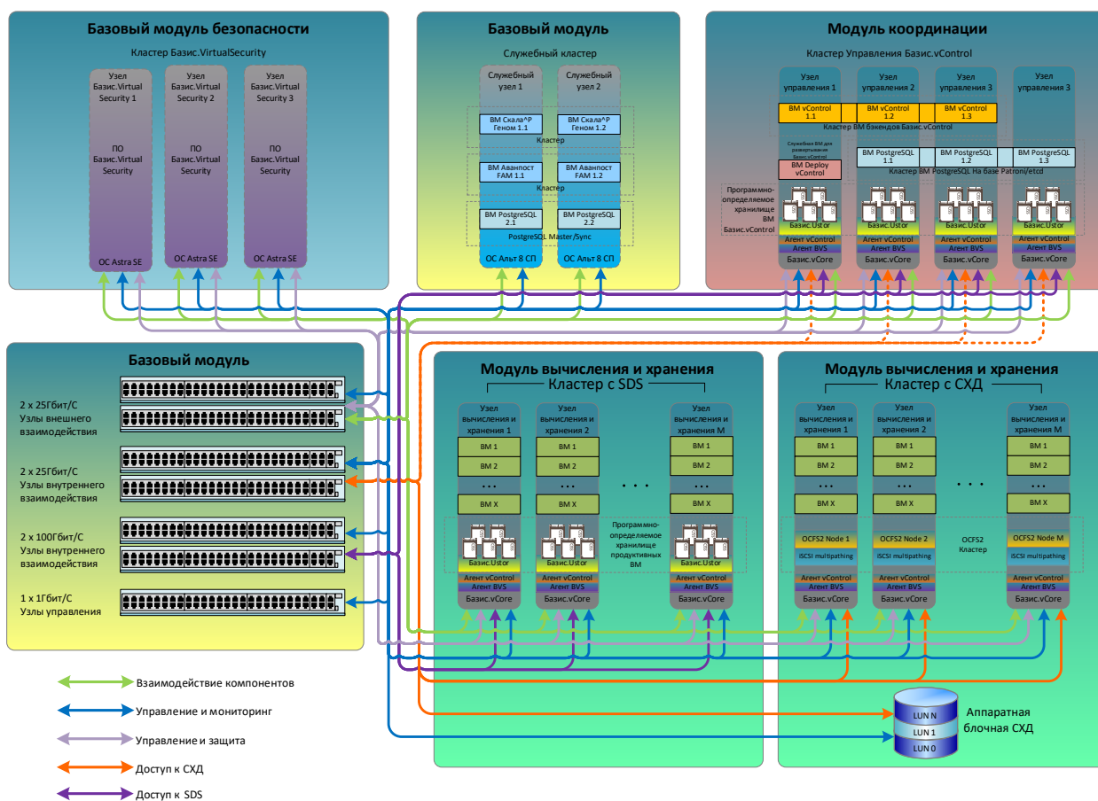
Рисунок 11. Узлы и программные компоненты в максимальной архитектуре Машины динамической инфраструктуры Скала^р МДИ.В
